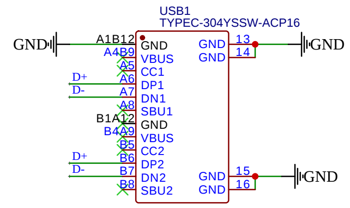
下载接口(仅下载不供电)
