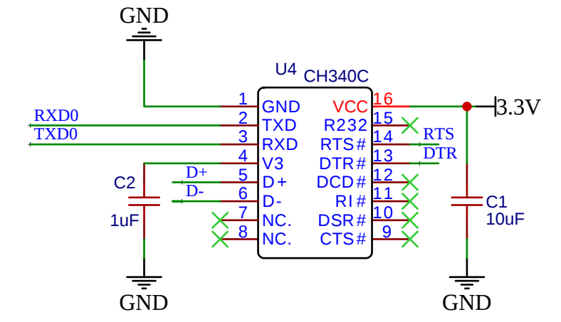
CH340 USB转串口
