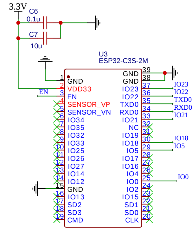
ESP32主控
